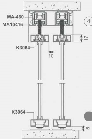
Двухрельсовая стандартная подвесная система + 2 двусторонних демпфера
