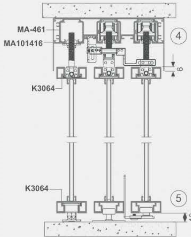
2+1 (три направляющие) Соединительный элемент для монтажа фиксированной створки + 2 синхронизированных подвижных створки + 1 двусторонний демпфер
