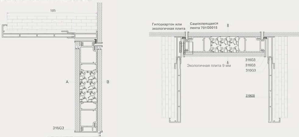
Схема сборки двойного комплекта скрыторамной алюминиево-деревянной экологичной распашной двери
