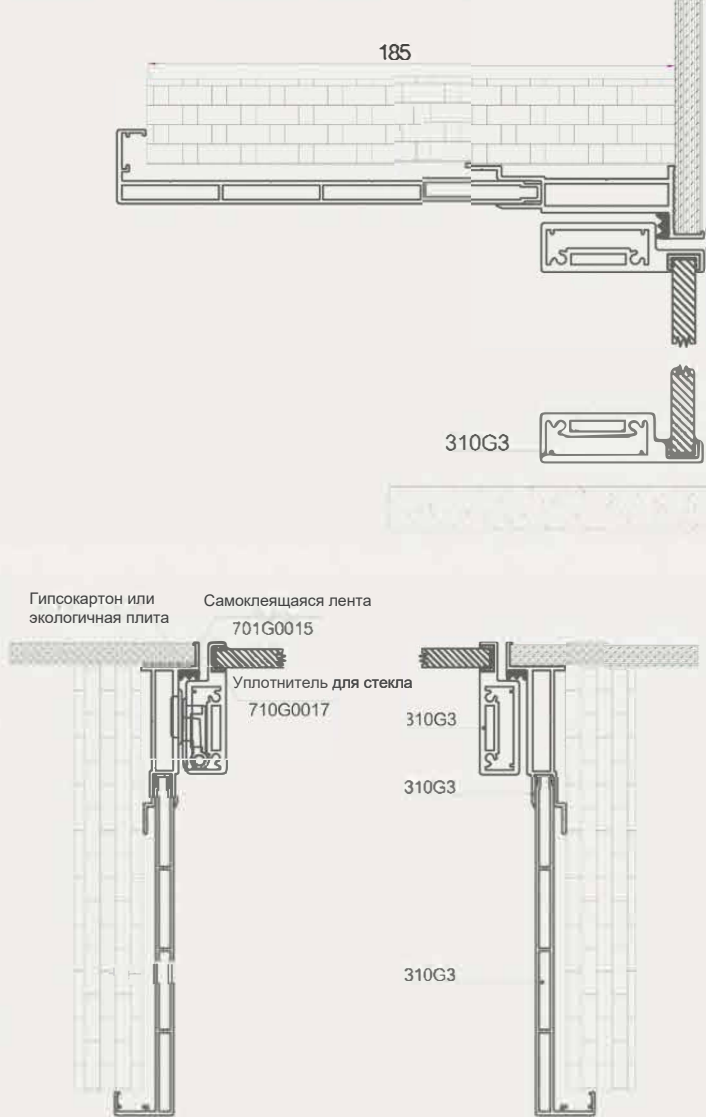
Схема сборки двойного комплекта скрыторамной распашной двери (стенная панель)
