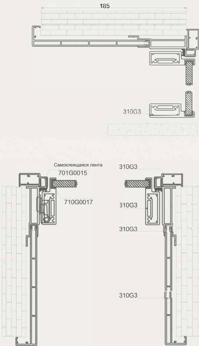
Схема сборки двойного комплекта скрыторамной распашной двери (алюминиевая дверная коробка)
