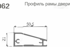
Профиль рамы двери
