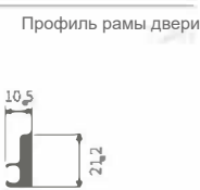
Профиль рамы двери
