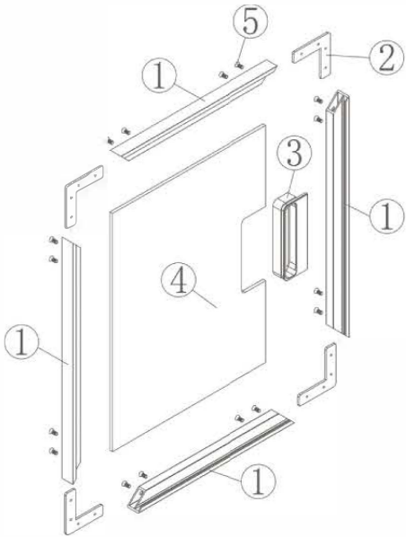
Профиль рамы двери
