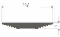
K3254 Внешний ползунок
