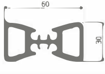
K3266 Передняя рама для наклонной полки
