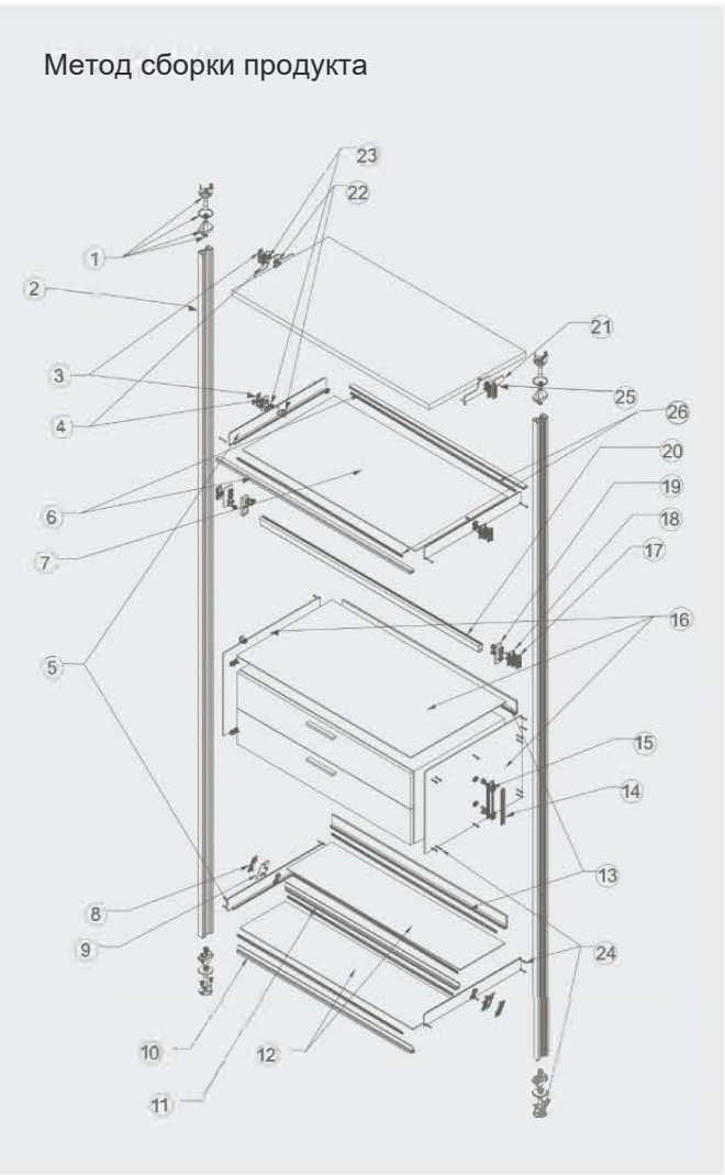
K3263 Боковая рама для стеклянной полки
